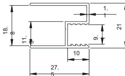
Profilo vetro
