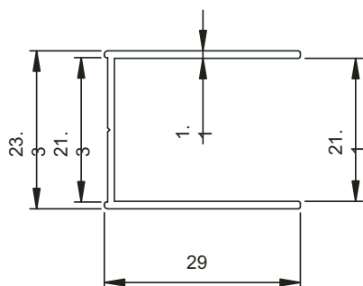
SEZIONE DEI PROFILI RAPID Profilo a muro
